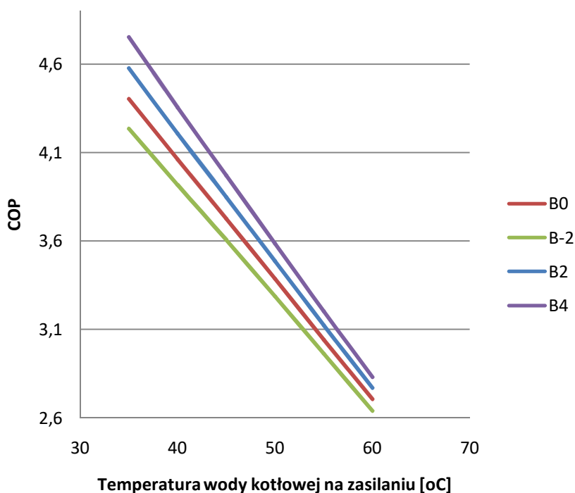
Zmienność COP od temp. D.Ż. przy 120Hz
