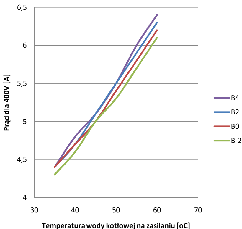
Prąd sprężarki od temp. D.Ż. przy 90Hz
