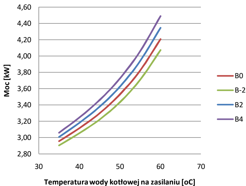
Zapotrzebowanie mocy wejściowej dla różnych temperatur dolnego źródła przy 120Hz
