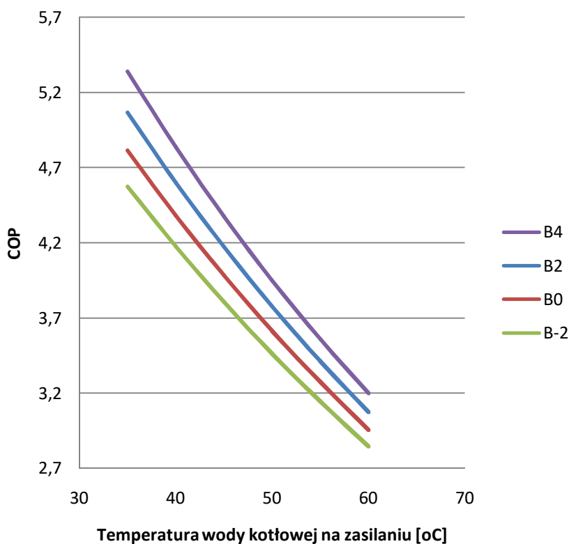
Zmienność COP od temp. D.Ż. przy 90Hz
