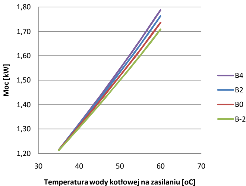
Zapotrzebowanie mocy wejściowej dla różnych temperatur dolnego źródła przy 60Hz
