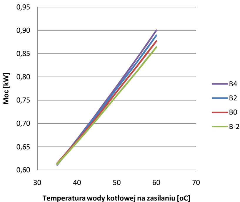
Zapotrzebowanie mocy wejściowej dla różnych temperatur dolnego źródła przy 30Hz
