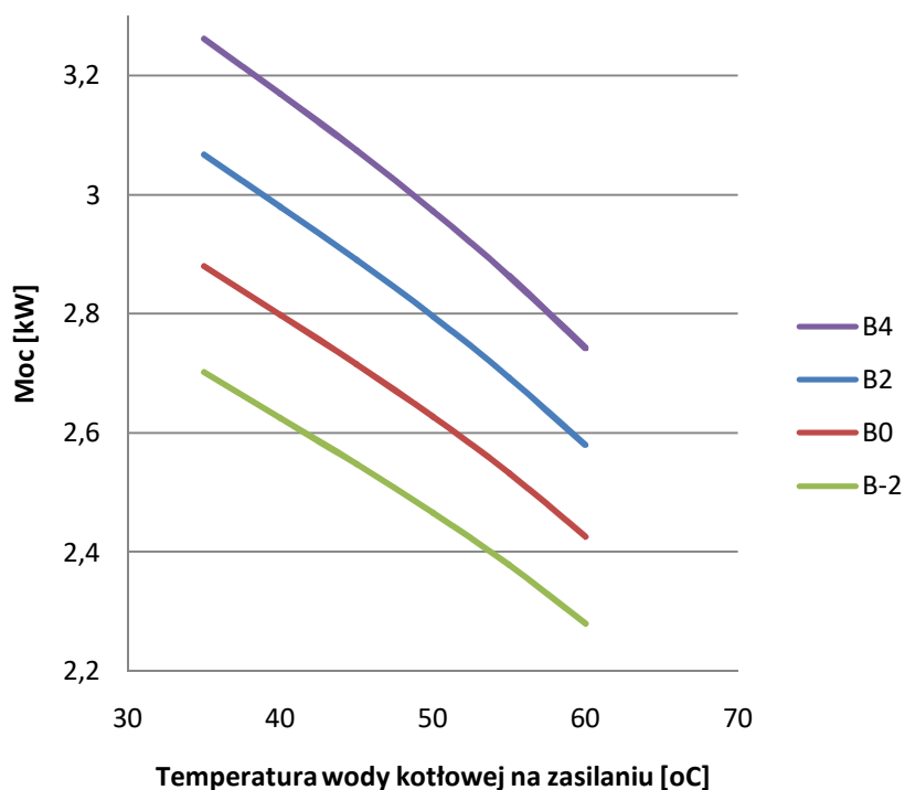
Moc grzewcza pompy ciepła od temp. D.Ż. przy 30Hz
