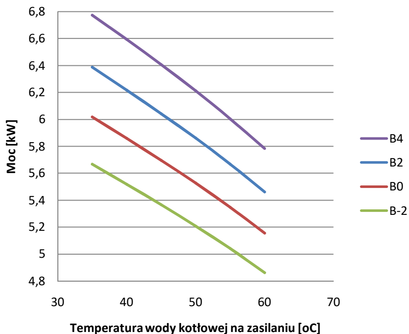
Moc grzewcza pompy ciepła od temp. D.Ż. przy 60Hz
