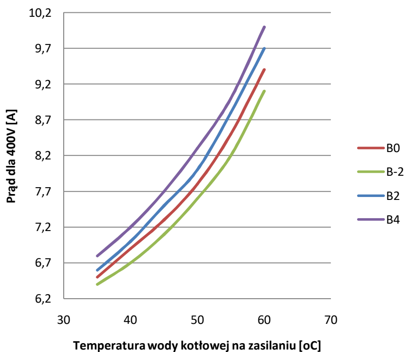
Prąd sprężarki od temp. D.Ż. przy 120Hz
